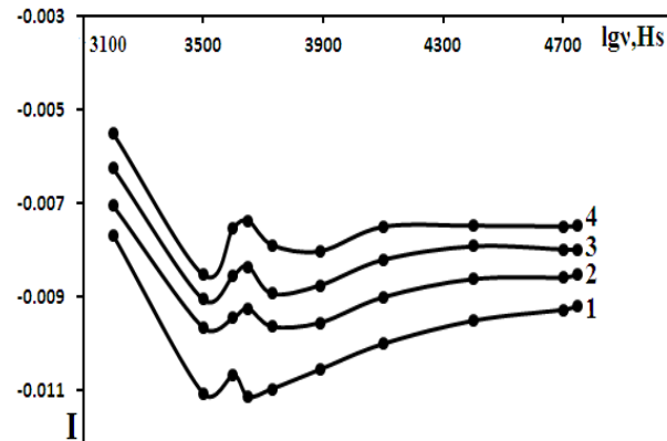
Şəkil 5. ASPE+xhəcm%Bi 2 Te 3 kompozitlərin elektrik enerji itkilərinin tezlikdən asılılıqları: 1-x=5; 2-x=10; 3-x=15; 4-x=20;
